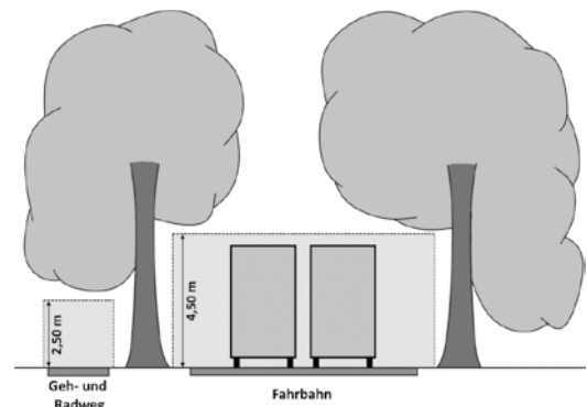
Lichtraumprofil: ast- und stammfreier Bereich (rot gekennzeichnet)
